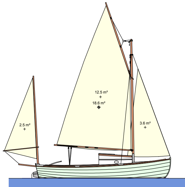
Option tape-cul à balestron
